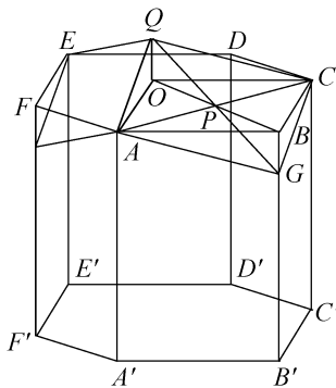
图 3.3.7 蜂房秘密
