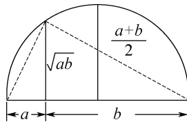
图 1.1.3 \sqrt{ab} < \frac{a+b}{2} 示意图
