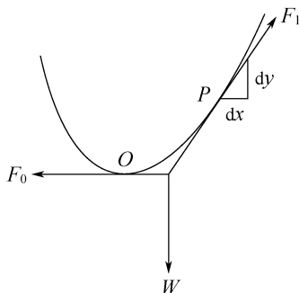
图 1.1.1 悬链线
